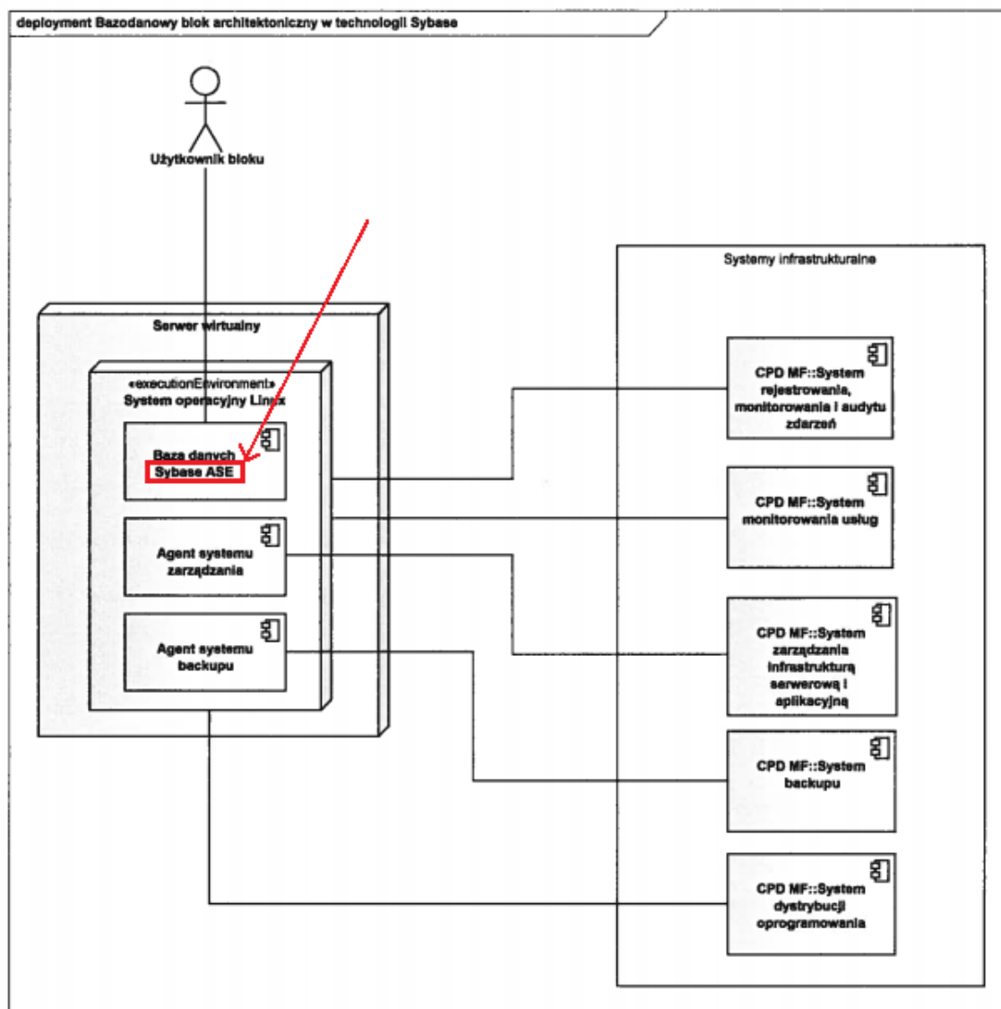
Rysunek 13 Model logiczny bloku architektonicznego B.DB.SYB
